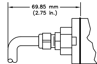
R Integral Cable
